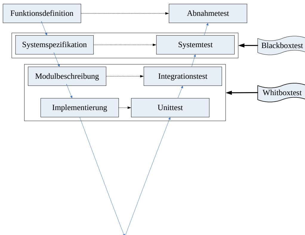
Abbildung 3: V-Modell
