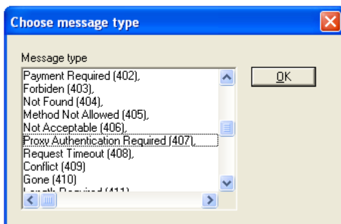
Abbildung 31: Messagetyp (407)
