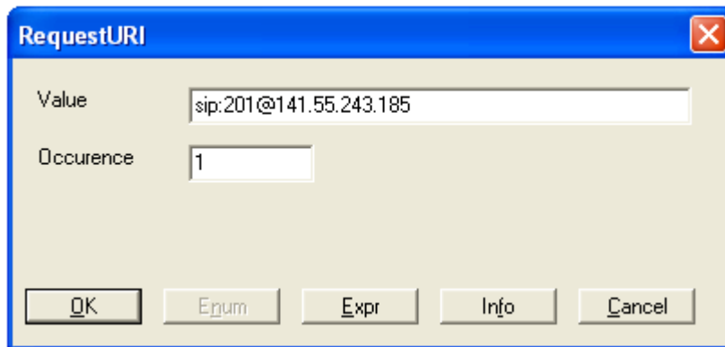
Abbildung 30: Request URI
