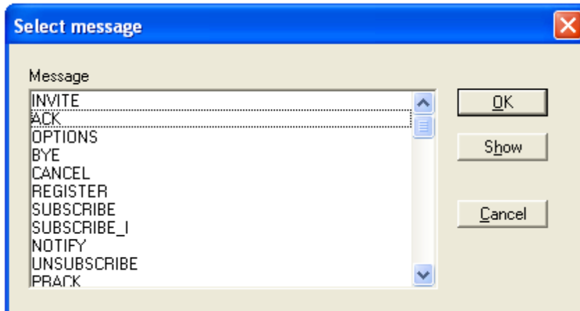
Abbildung 32: Nachricht auswählen
