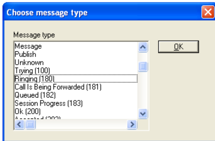
Abbildung 33: Messagetyp (180)
