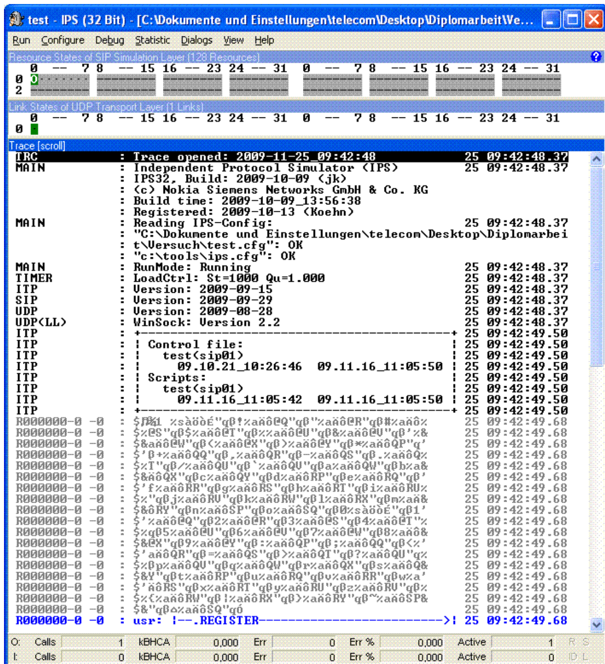
Abbildung 4: IPS-Fenster
