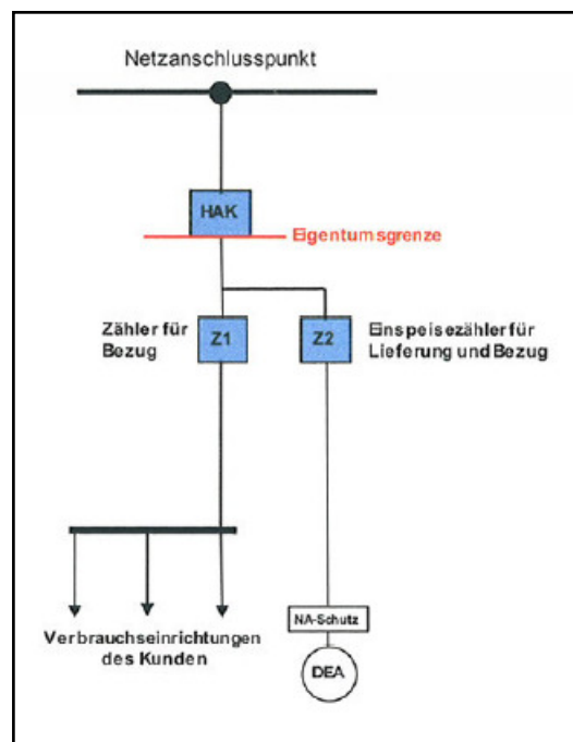
Abb. 1-1: Aufbau der Photovoltaikanlage mit 2 Zählern
