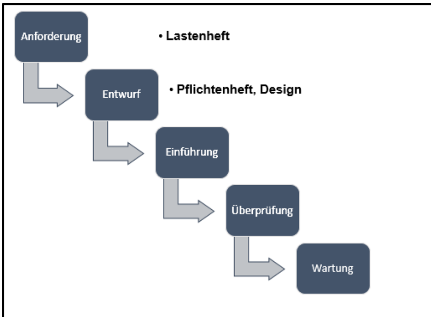
Abb. 1: Wasserfallmodell
