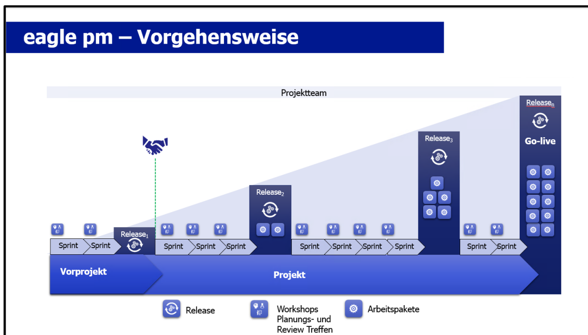
Abb. 13: Vorgangsweise eagle
